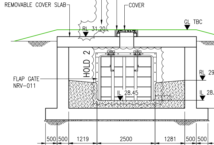
SECTION 2 SCALE: 1:50
